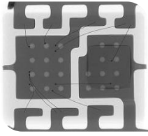
IC wire
